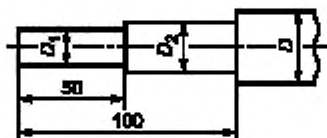
Рисунок А.1 — Форма образца
